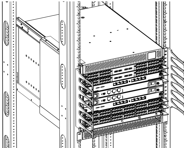
FIGURE 5 Systèmes de doigts de passage de câbles verticaux
