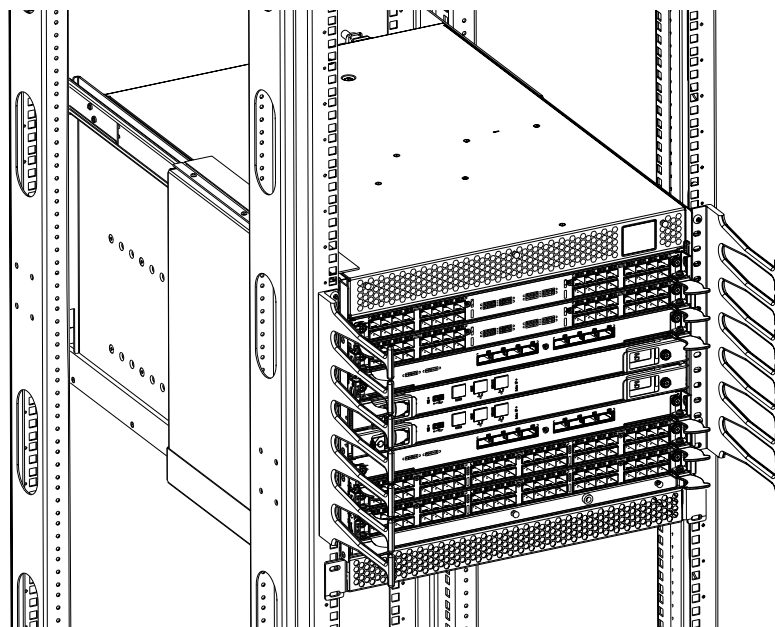
FIGURA 5 Conjuntos das linguetas de gerenciamento de cabos
