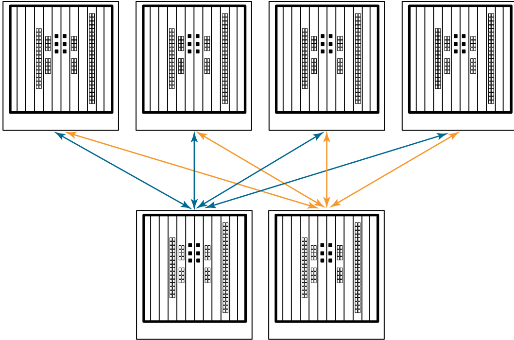
그림 9 DCX 8510 코어 / 에지 ICL 토폴로지
