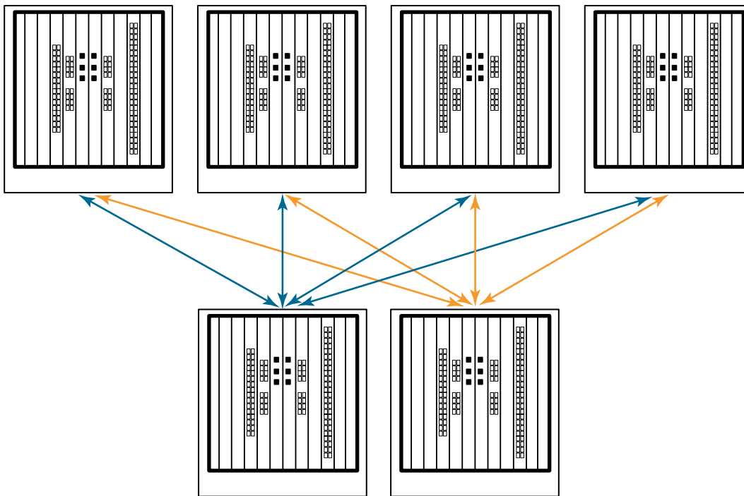
ILUSTRACIÓN 9 Topología ICL central o perimetral DCX 8510
