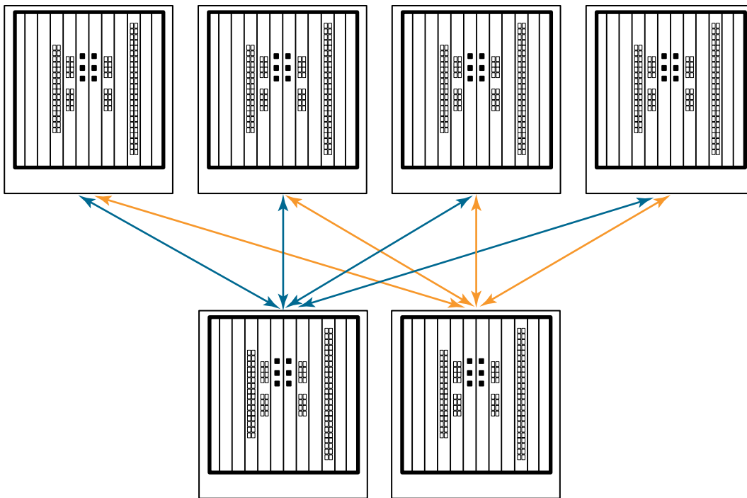
FIGURA 9 Topologia ICL núcleo/borda DCX 8510
