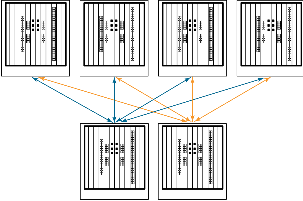
ŞEKİL 9 DCX 8510 çekirdek/kenar ICL topolojisi
