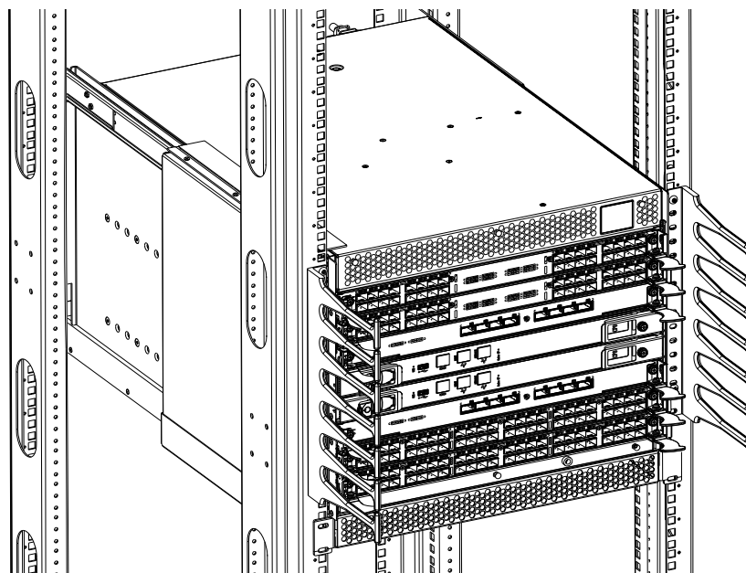
איור 5 מכלולי אצבעות אנכיות לניהול כבלים
