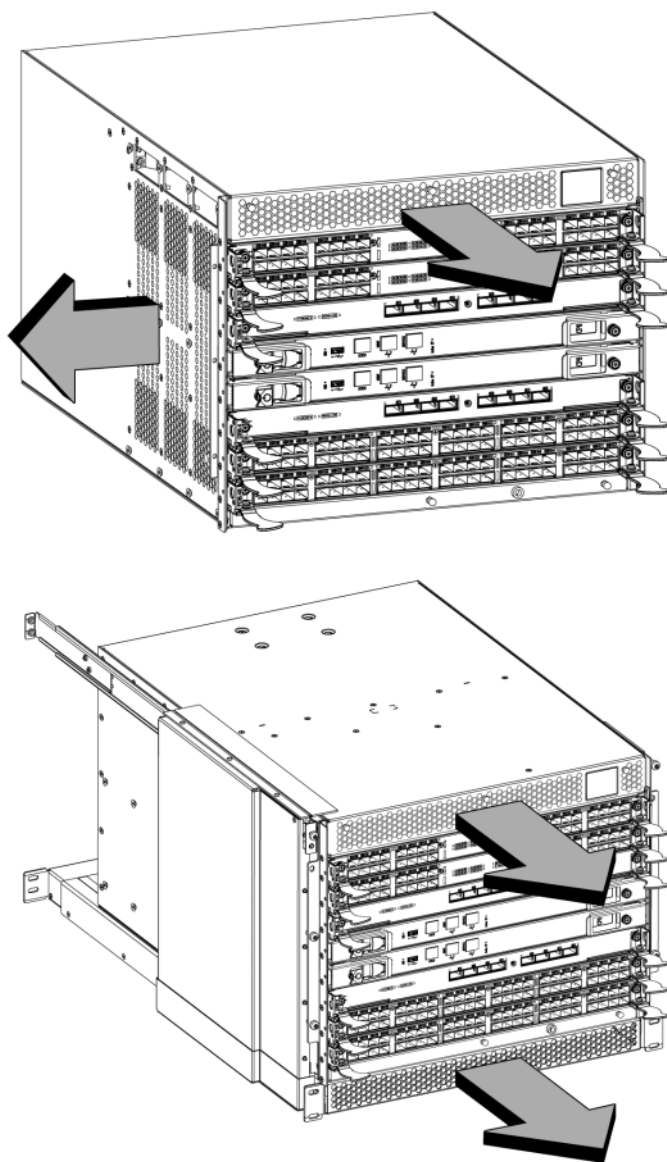
FIGURA 3 Comparação do fluxo de ar do Brocade DCX 8510-4 sem (acima) e com (abaixo) o kit de exaustão do lado das portas instalado (exemplo de configuração)
