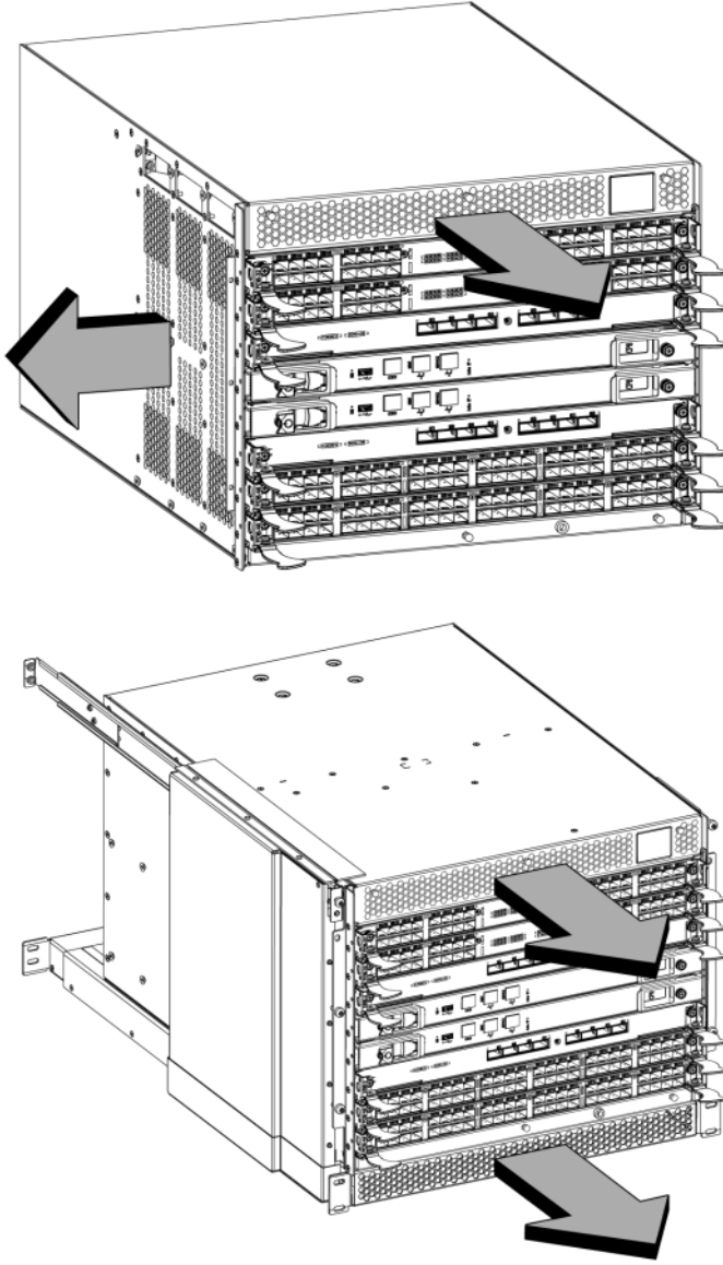
ŞEKİL 3 Bağlantı noktası tarafı hava çıkış kiti monte edilmemiş ve edilmiş iki Brocade DCX 8510-4 ürünündeki hava akışının karşılaştırılması (örnek yapılandırma)
