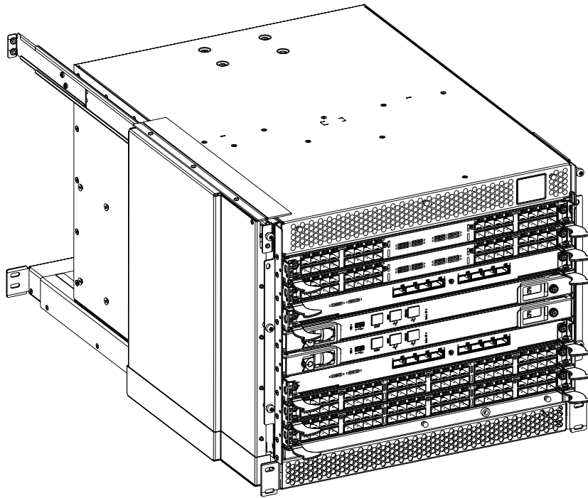
GAMBAR 2 Sisi port Brocade DCX 8510-4 dengan kit pembuangan sisi port yang sudah terpasang (konfigurasi sampel)
