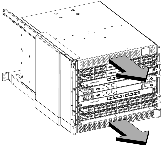
איור 3 השוואת זרימת אוויר של ה- Brocade DCX 8510-4 ללא ערכת Port Side Exhaust ועם ערכה מותקנת (תצורה לדוגמה)
