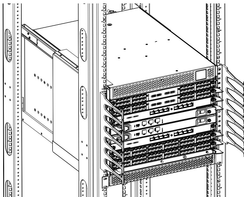
図 5 垂直型ケーブル管理フィンガーアセンブリ
