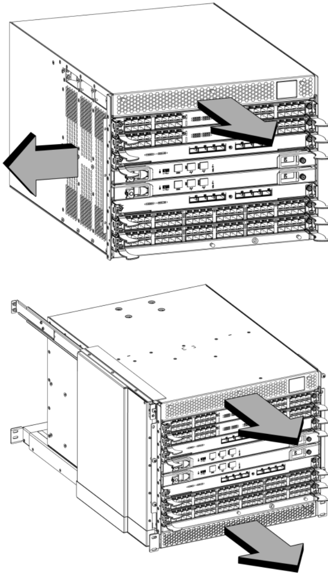
圖 3 Brocade DCX 8510-4 有（下圖）、無（上圖）安裝連接埠側邊排氣套件的氣流比較（設定樣本）
