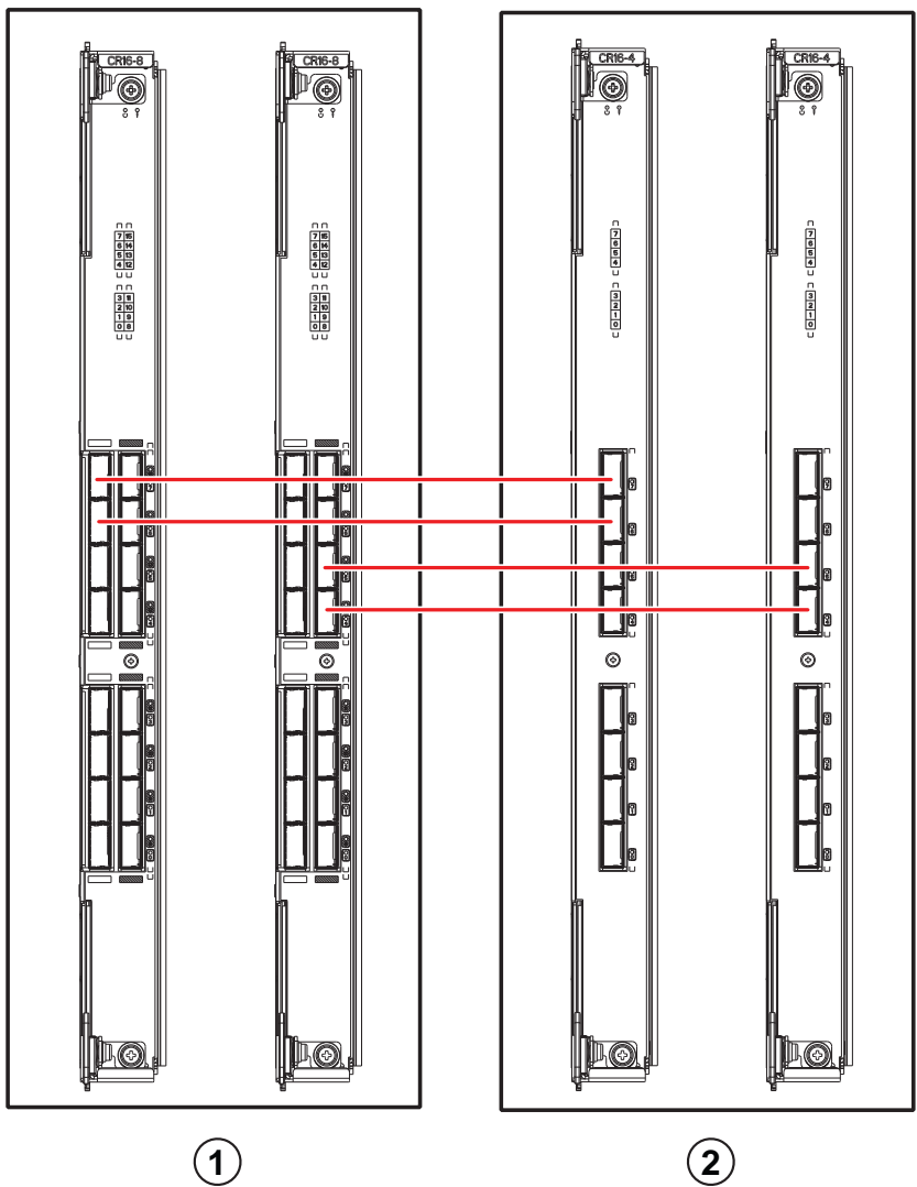
FIGURE 8 Branchement des câbles QSFP – exemple de configuration 8510 - type parallèle
