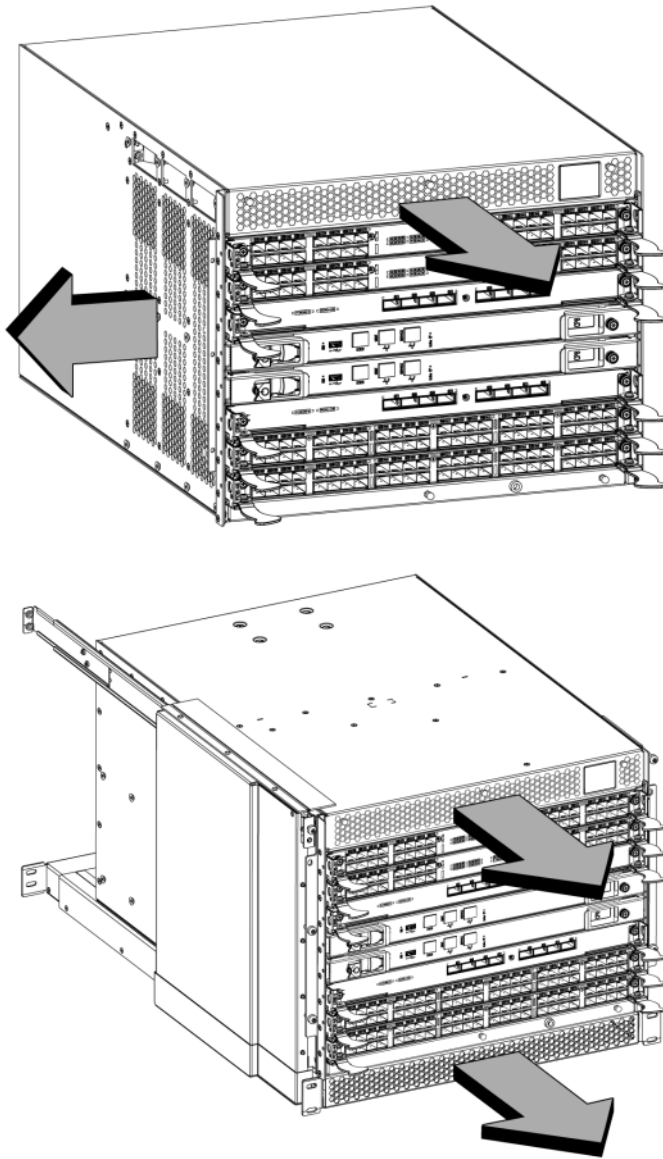
図 3 Brocade DCX 8510-4 にポート側排気キット未設置（上記）時と、設置時（下記）におけるエアフローの比較（サンプル構成）
