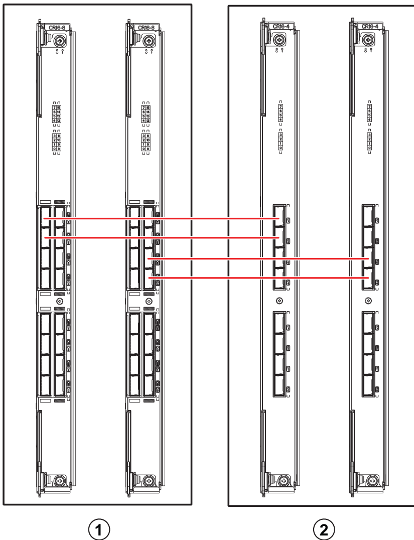
FIGURA 8 Conexões de cabos QSFP (Quad Small Form-factor Pluggable) – amostra de configuração do 8510 – conexão paralela
