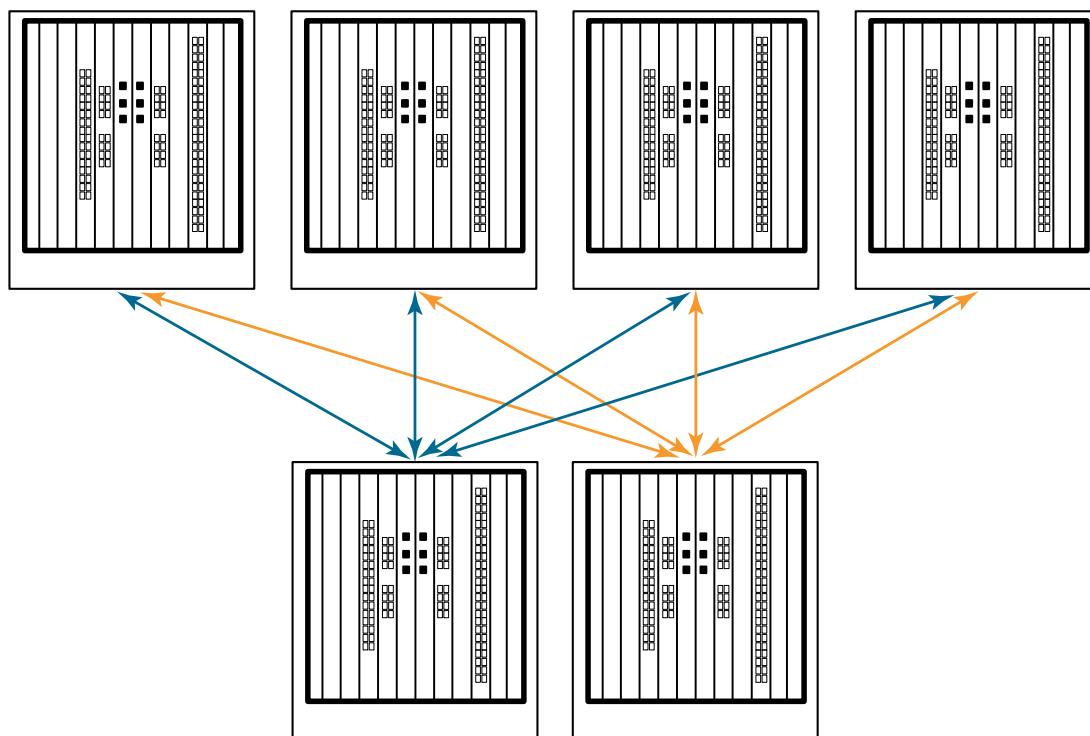
איור 9 טופולוגיית LCL מסוג ליבה/להב DCX 8510
