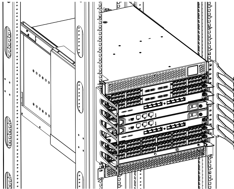
그림 5 수직 케이블 관리 핑거 조립품
