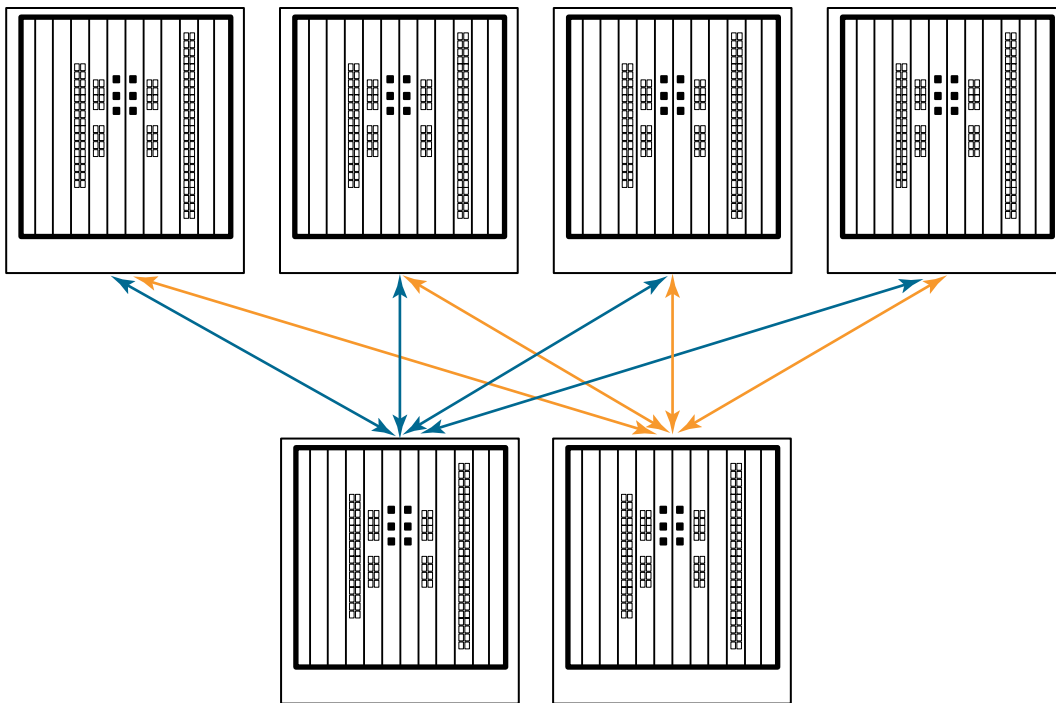
圖 9 DCX 8510 核心／邊緣 ICL 拓樸
