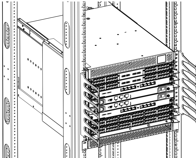
ILUSTRACIÓN 5 Ensamblajes para la administración de cables vertical
